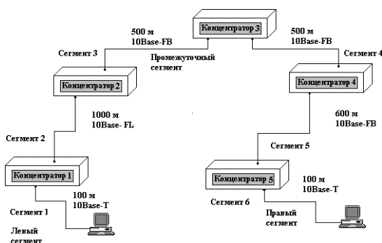
Рисунок 1. Пример сети Ethernet
