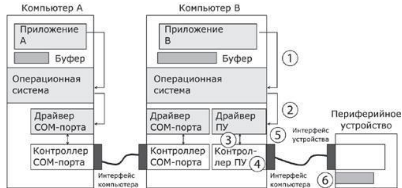
Рис. 2. Взаимодействие двух компьютеров.
