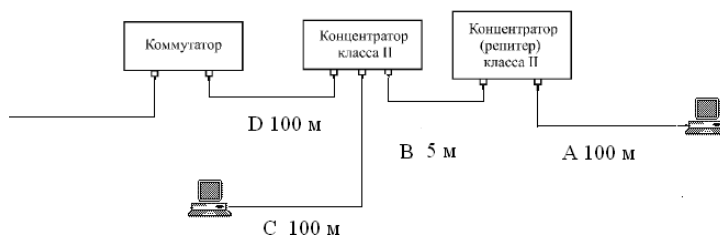
Рисунок 5. Пример максимальной конфигурации сети Fast Ethernet
